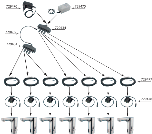
EXAMPLE OF MULTIPLE INSTALLATION - ESEMPIO DI INSTALLAZIONE MULTIPLA - EXEMPLE D'INSTALLATION MULTIPLE - BEISPIEL FÜR EINE MEHRFACHINSTALLATION - EJEMPLO DE INSTALACIÓN MÚLTIPLE
