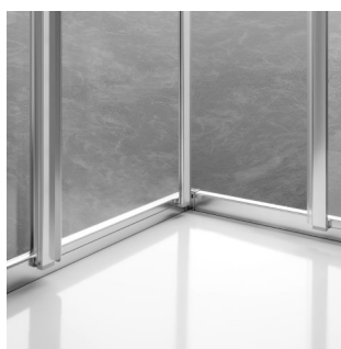
Bodenprofil magnetgeführt
