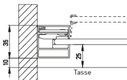
Modde 1: Montage auf Tasse
