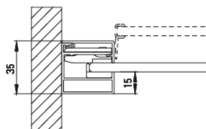
Modde 1: bodenebene Montage
